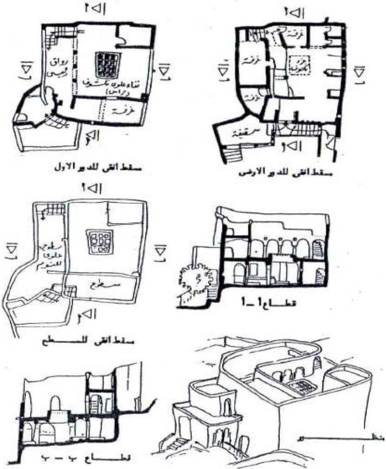
(شكل 71) نموذج للمسكن التقليدي بوادي مزاب في صحراء الشبكة بالجزائر عن وائل حسين: نفس المرجع، شكل 4
