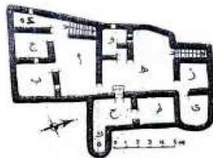
(شكل 65) مسقط أفقي للدور الأرضي بدار بيلدة بلات عن: سعد شهاب: نفس المرجع، شكل 40
