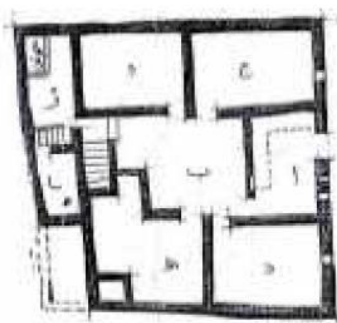
(شكل 66) مسقط أفقي للدور الأرضي بدار بيلدة تسالي عن: سعد شهاب: نفس المرجع، شكل 72
