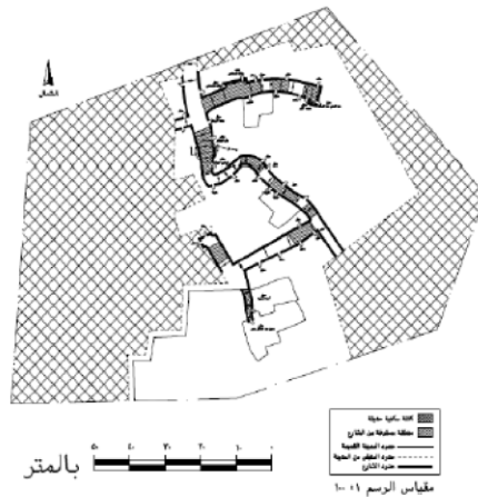
(خريطة 5) الأجزاء الباقية من درب السندانة بالخارجة عمل الباحث
